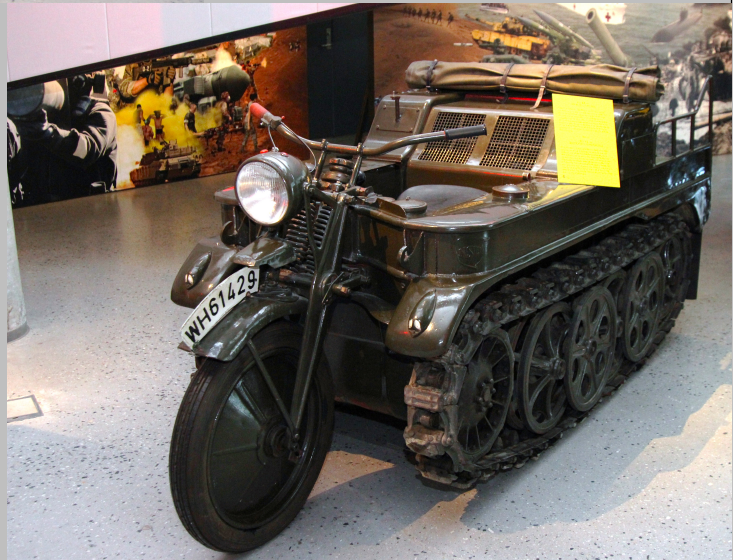
Høyre: "Tysk beltemotorsykel med 36 hk Opelmotor. 6 gir forover 2 revers. Vekt 1350 kg» «Kettenkrad»
